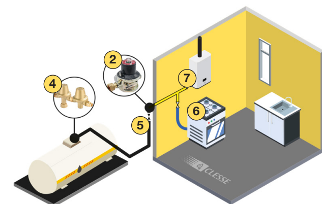
CITERNE - 1er étage + 2ème étage DSI
