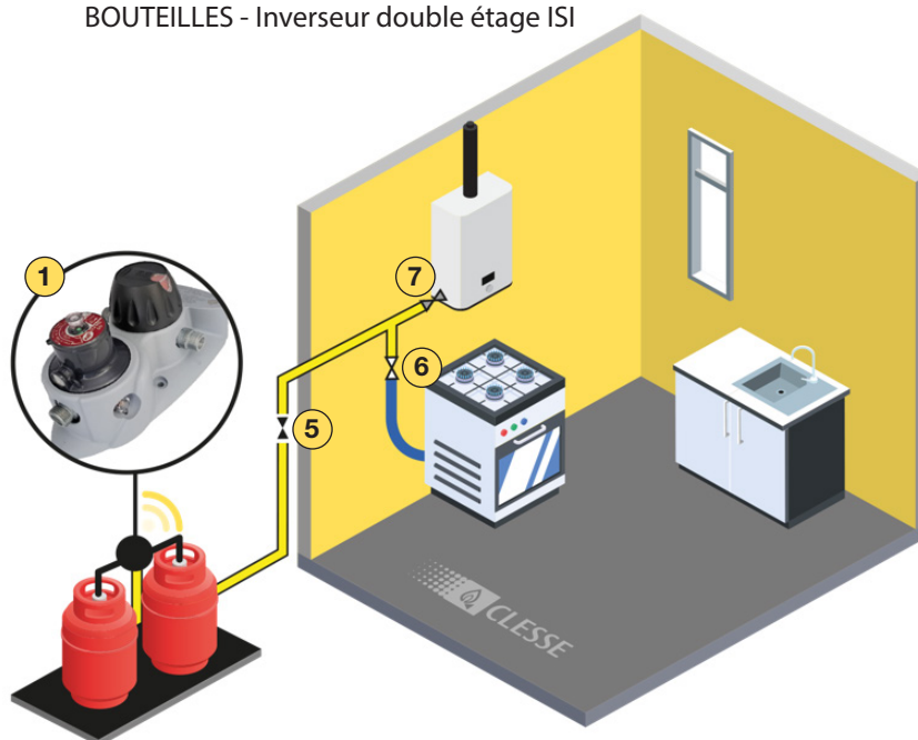
BOUEILLES - 1er étage 2175 + 2ème étage DSI
