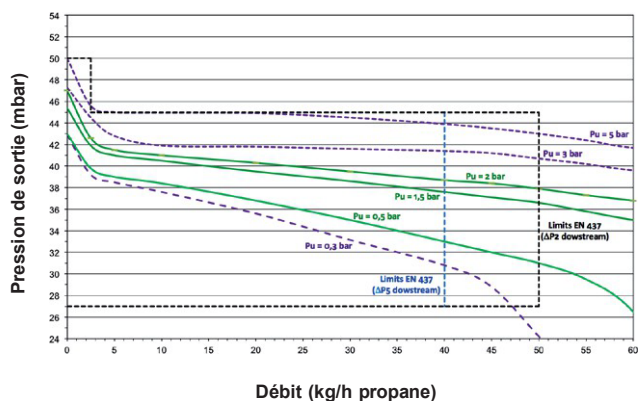
BP2403 – Réglage 37 mbar selon EN 16129 et EN 437
