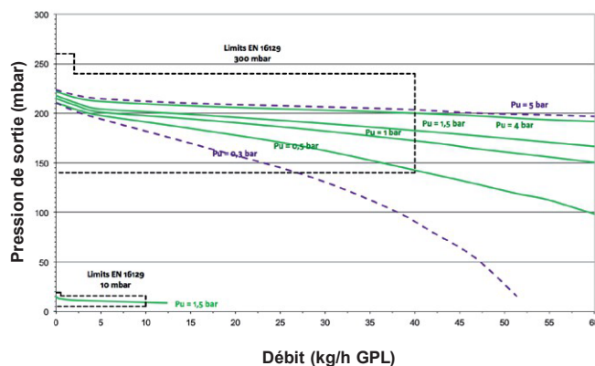
BP2403R - Réglable de 10 à 200 mbar selon EN 16129
