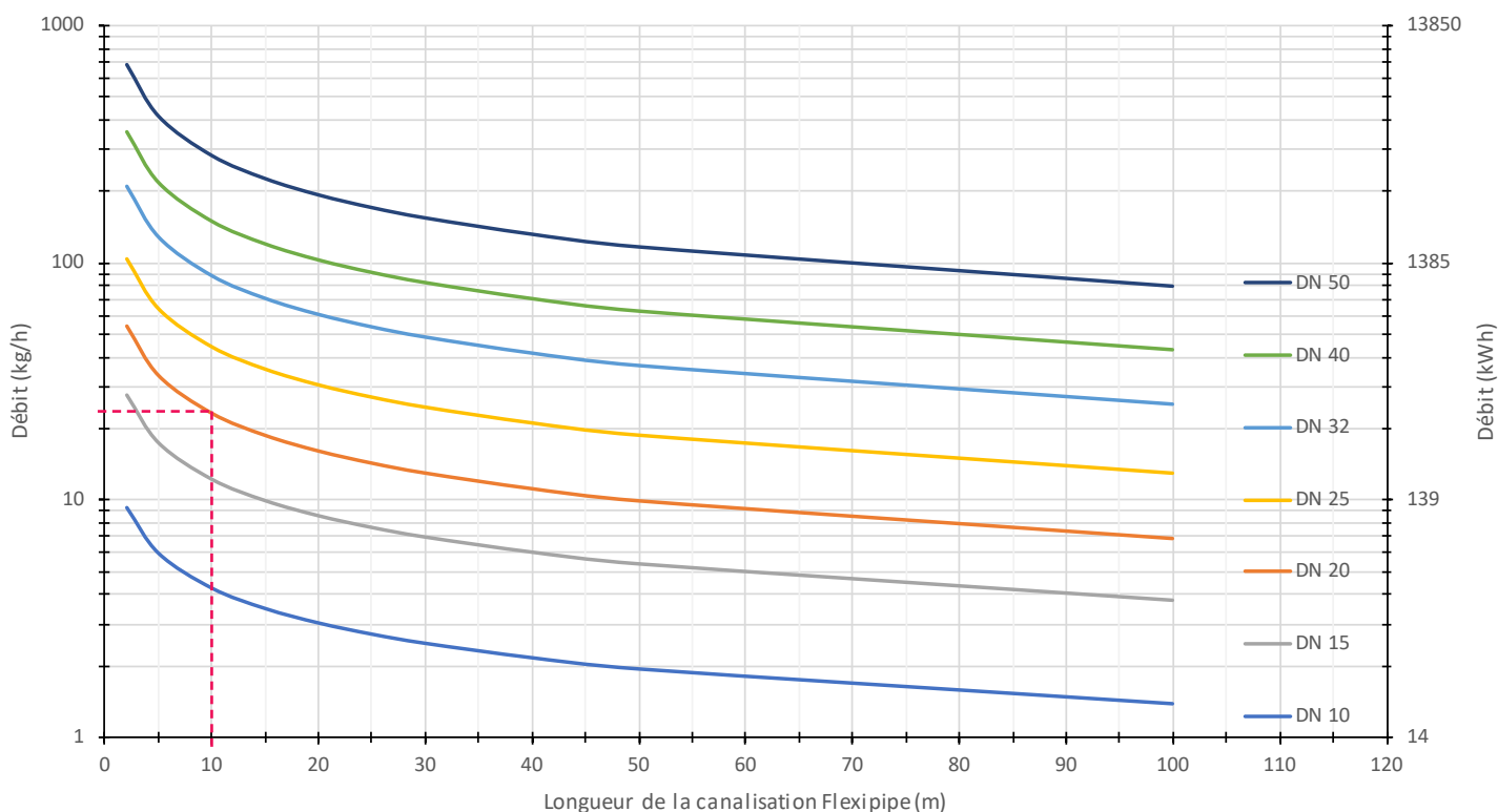
Capacité de débit Propane 300 mbar - \Delta P 10%
