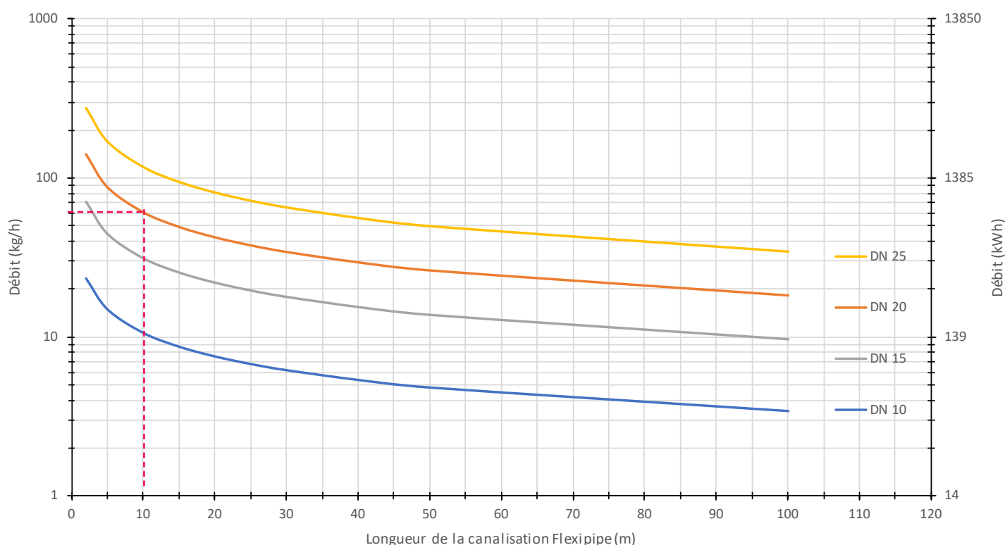
Capacité de débit Propane 1,5 bar - \Delta P 150 mbar
